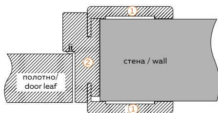
Схема монтажа без использования добора Adjustable door frame
